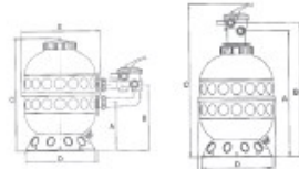
Dimensions du filtre HI Side
