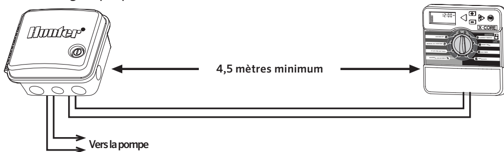
Relais démarrage de pompe
